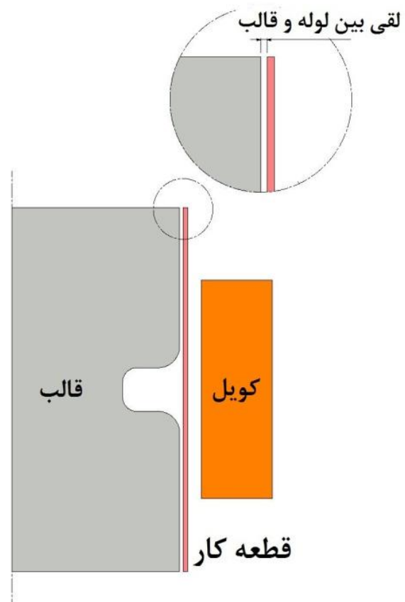
شکل (۵): شماتیک قطعه کار، سیم‌پیچ و قالب به صورت تقارن محوری در فرایند تراکم لوله.
